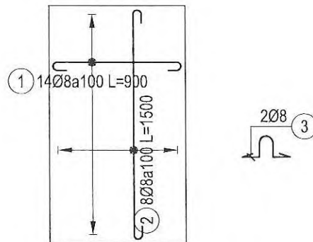
MẶT BẰNG TẤM ĐAN (SL=2)
