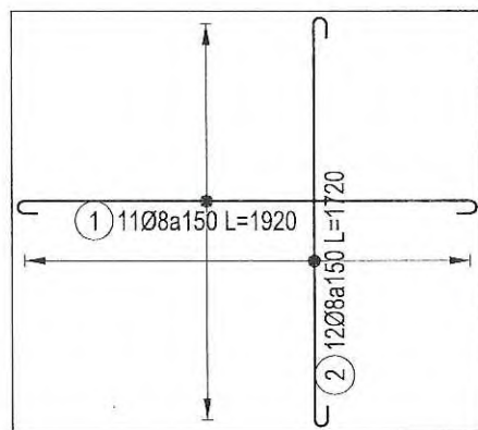
MẶT BẰNG THÉP DÂY BÊ (SL=1)
