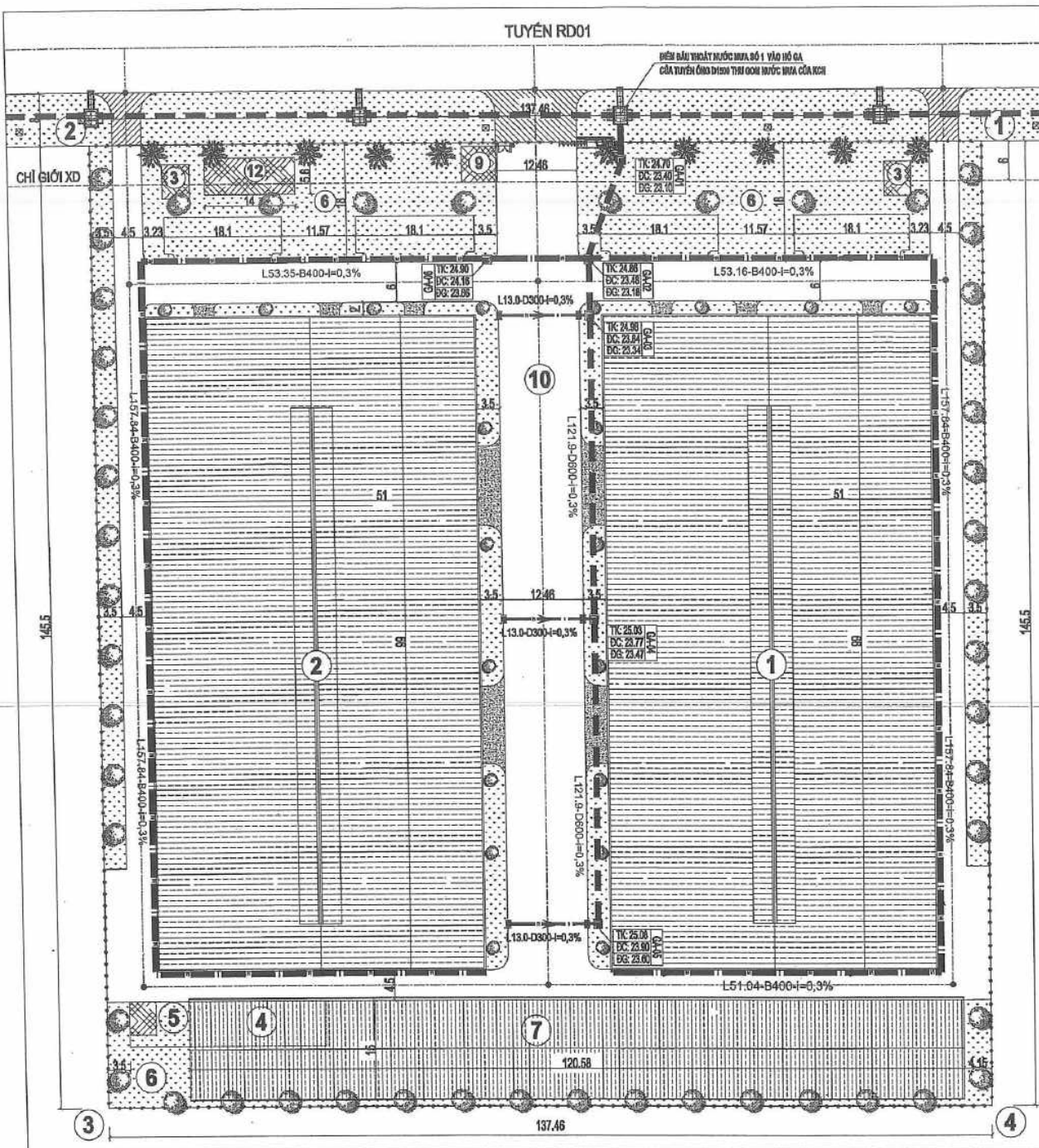
MẶT BẰNG THOÁT NƯỚC MƯA
