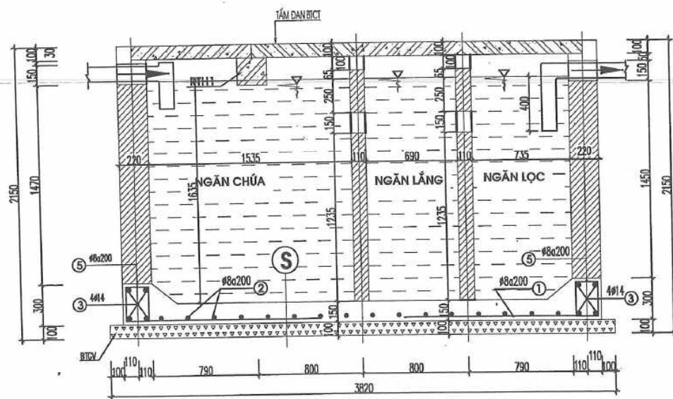
MẶT CẮT 1-1
