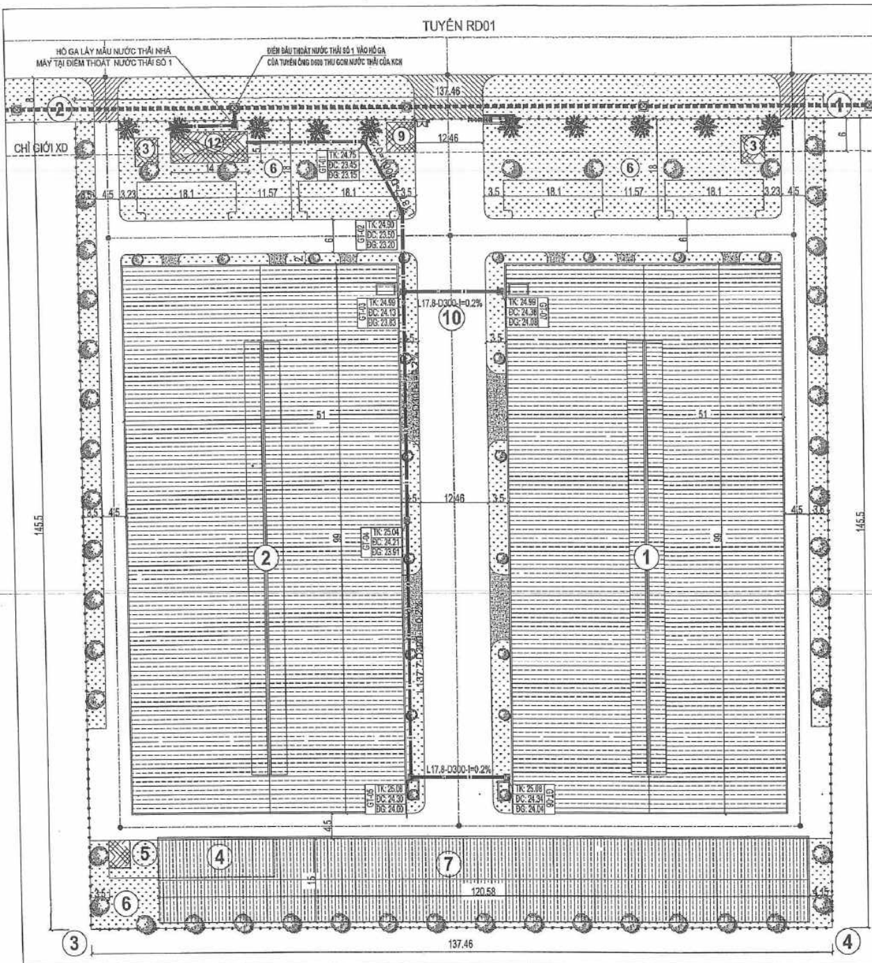
MẶT BẰNG THOÁT NƯỚC THẢI
