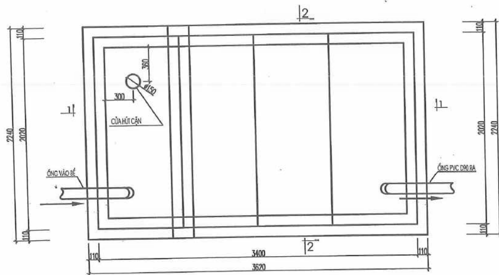
MẶT BẰNG BÊ TỰ HOẠI SL:02
