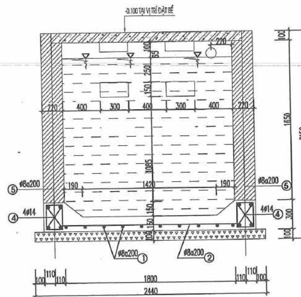
MẶT CẮT 2-2
