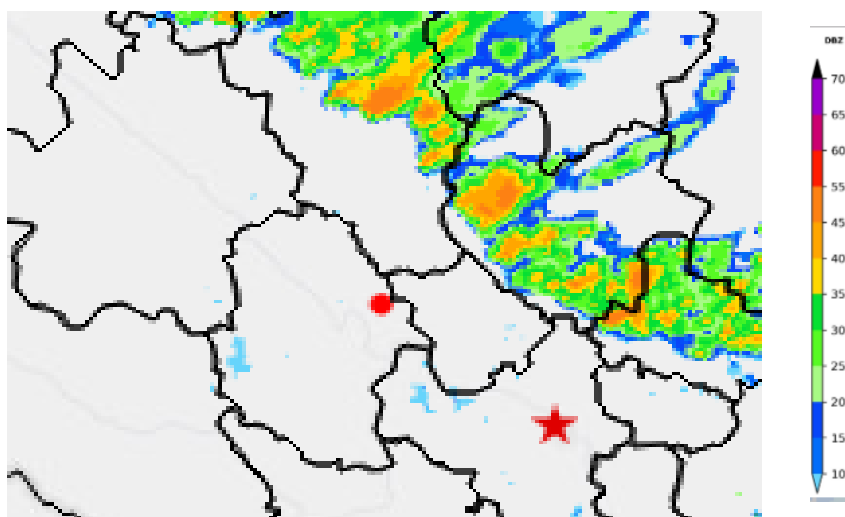
Hình 1: Ảnh radar thời tiết tỉnh Phú Thọ
